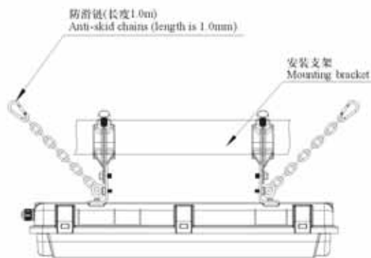
支架式安装 Bracket type
